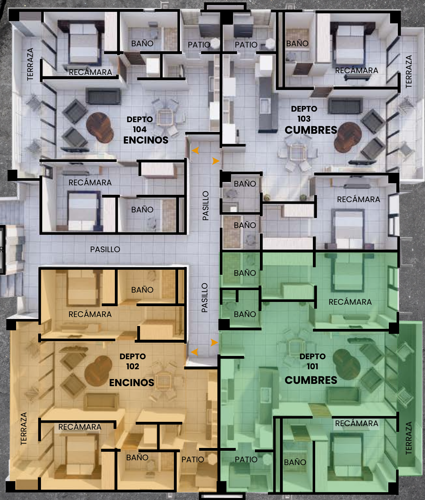
PLANTA ARQUITECTÓNICA TIPO PARA NIVEL 1, 2, 3 Y 4
